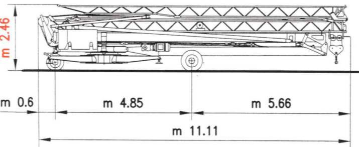
GRU IN TRASPORTO CON ZAVORRA DI MONTAGGIO
