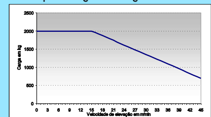
DIAGRAMA DE VELOCIDADE / Speed Diagram / Diagrama de Velocidad
